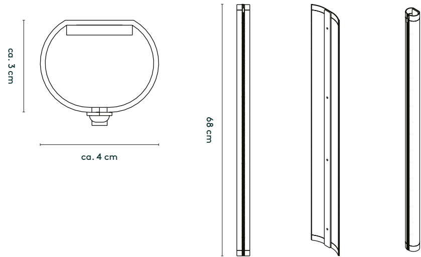
(Zip) cable channel
